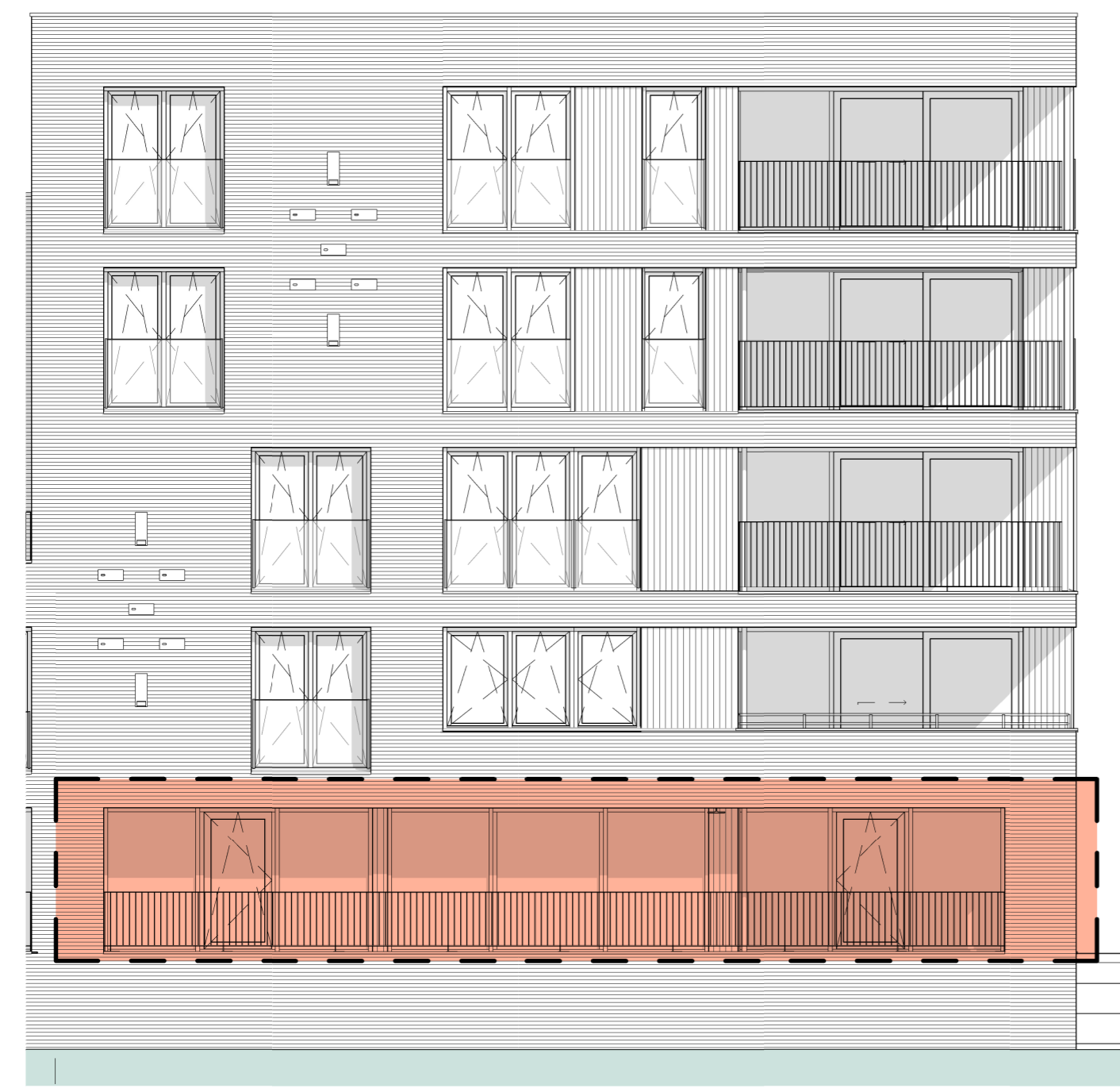
Gevel zuidzijde
